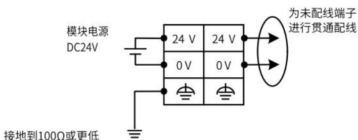
图 3-1 连接 FA7500 的系统电源
