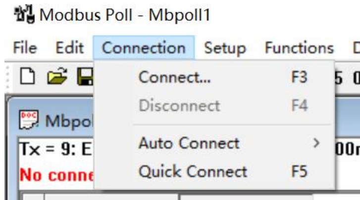
图 5.1 Connection 设置
