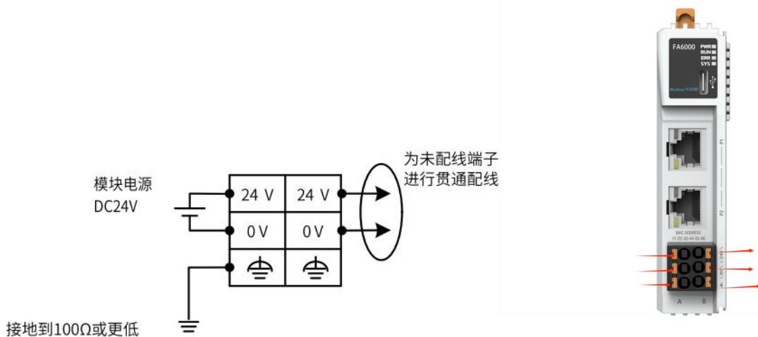
图 3-1 连接 FA6000 的系统电源
